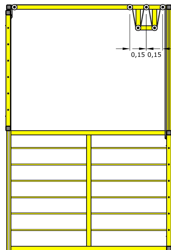
Corte AA Esc: 1/20
