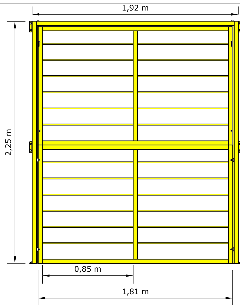
Frontal Esc: 1/20
