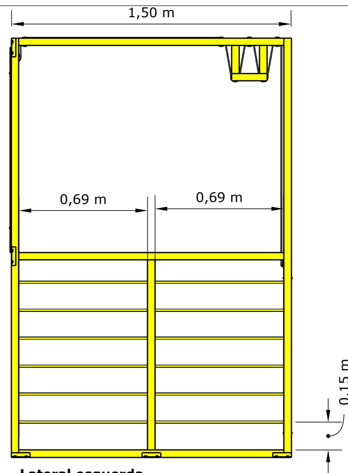
Lateral esquerda Esc: 1/20
