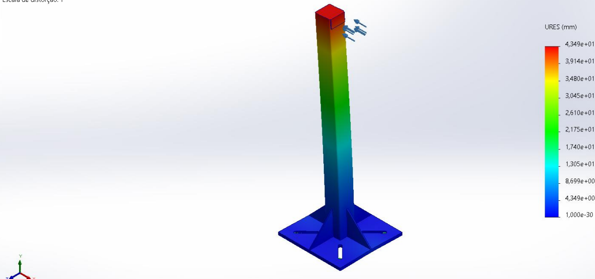
Peça2-Análise estática 1-Deslocamento-Deslocamento1
