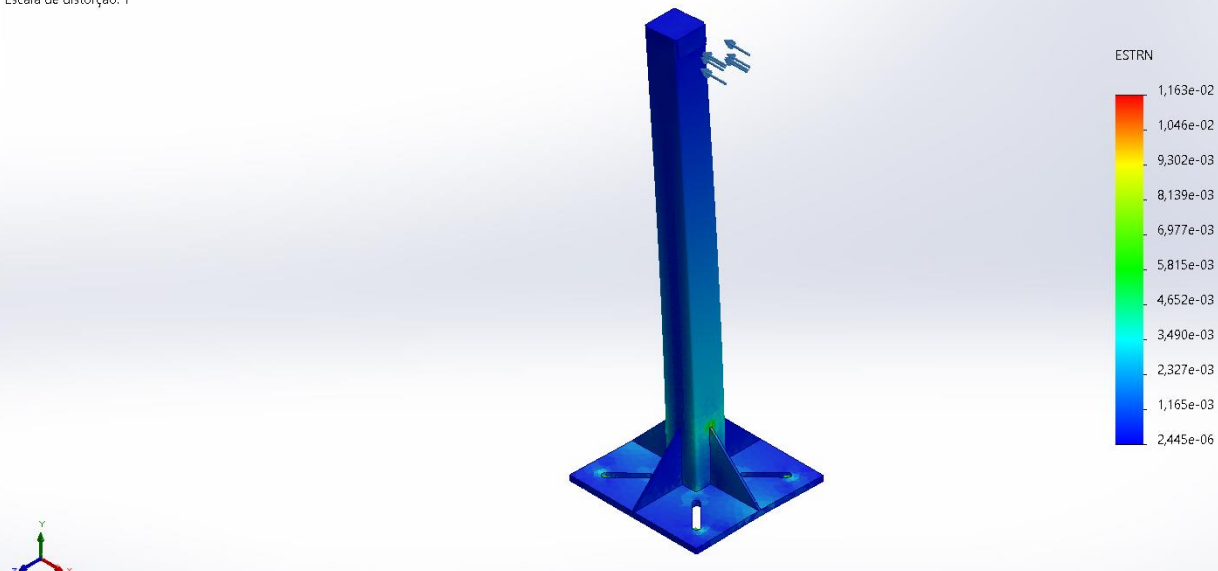
Peça2-Análise estática 1-Deformação-Deformação1
